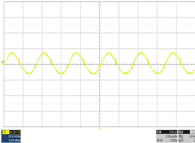
Noise V_{IN}=24V , I_O=12.5A , 20MHz Bandwidth
