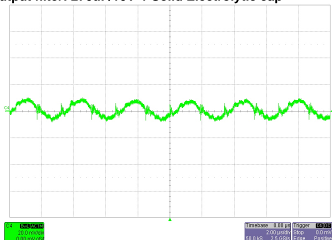
Noise V_{IN}=24V , I_O=24A , 20MHz Bandwidth
