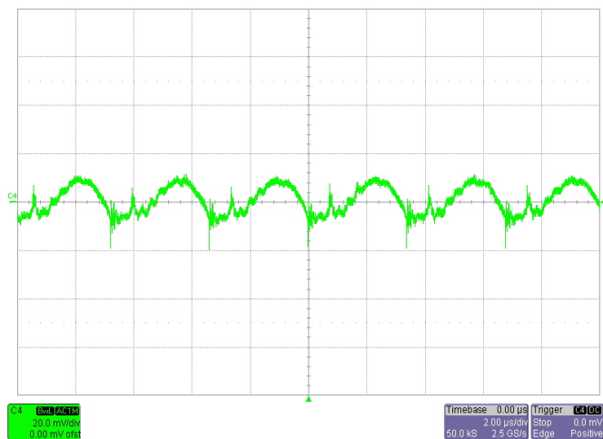
Noise V_{IN}=48V , I_O=24A , 20MHz Bandwidth
