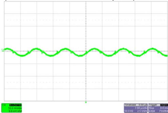
Noise V_{IN}=24V , I_O=10A , 20MHz Bandwidth
