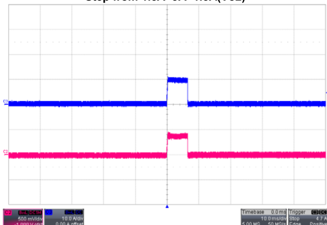
Short-Circuit Output VIN=12V(Vo2)
