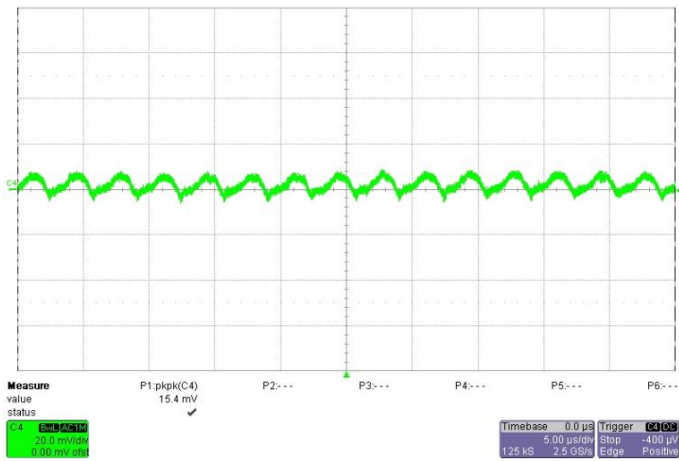
Noise V_{IN}=12V , I_O=8A , 5~20MHz Bandwidth
