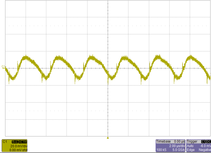
Noise V_{IN}=5.0V , I_O=30A , 5~20MHz Bandwidth
