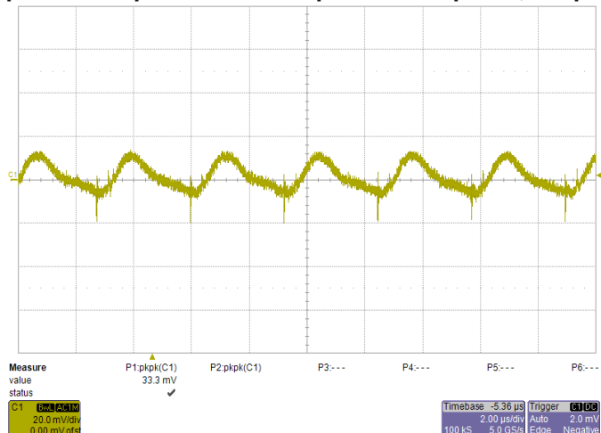
Noise V_{IN}=12V , I_O=26A , 5~20MHz Bandwidth
