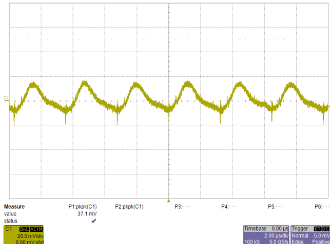
Noise V_{IN}=12V , I_O=26A , 5~20MHz Bandwidth
