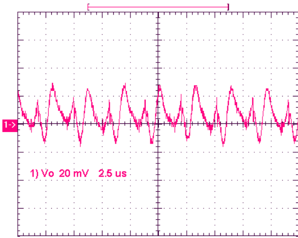
Noise V_{IN}=12V , I_O=16A , 5~20MHz Bandwidth
