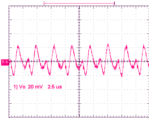
Noise V_{IN}=12V , I_O=16A , 5~20MHz Bandwidth
