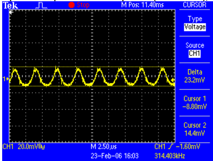
Noise V_{IN}=5V , I_O=20A , 5–20MHz Bandwidth
