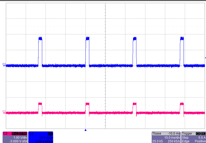
Short-Circuit Output V_{IN}=4.5V
