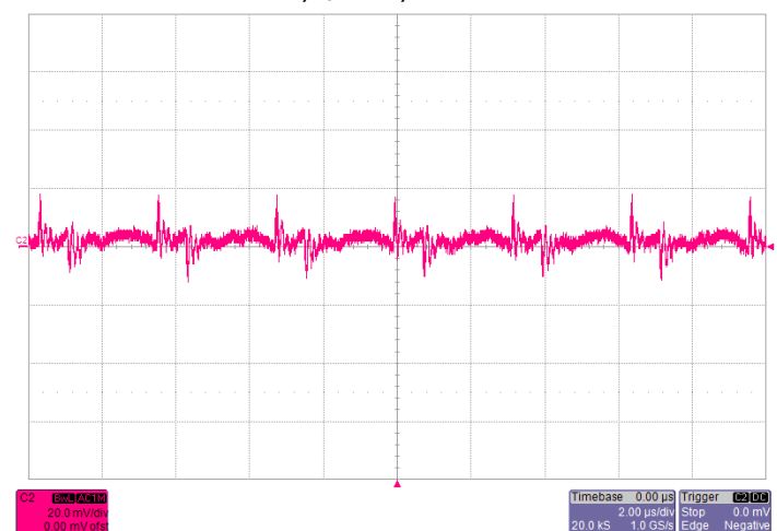
Noise V_{IN}=5.5V , I_O=10A , 5~20MHz Bandwidth
