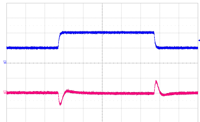
Noise V_{IN}=5.5V , I_O=10A , 5~20MHz Bandwidth
