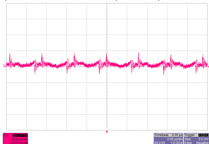
Noise V_{IN}=4.5V , I_O=10A , 5~20MHz Bandwidth
