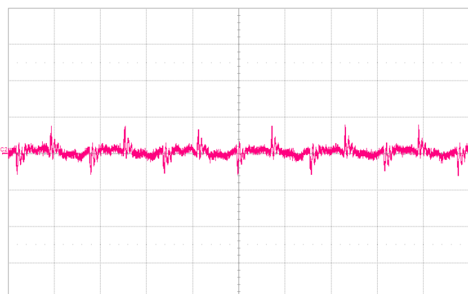
Noise V_{IN}=5V , I_O=10A , 5~20MHz Bandwidth
