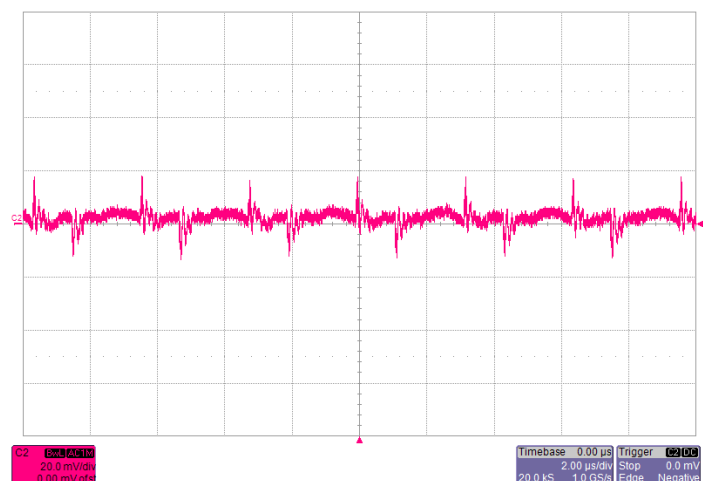
Noise V_{IN}=5.5V , I_O=10A , 5~20MHz Bandwidth
