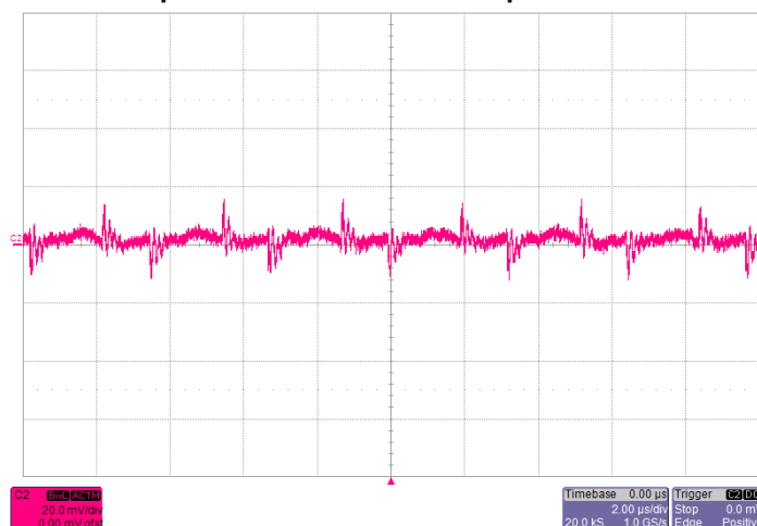
Noise V_{IN}=5V , I_O=10A , 5~20MHz Bandwidth
