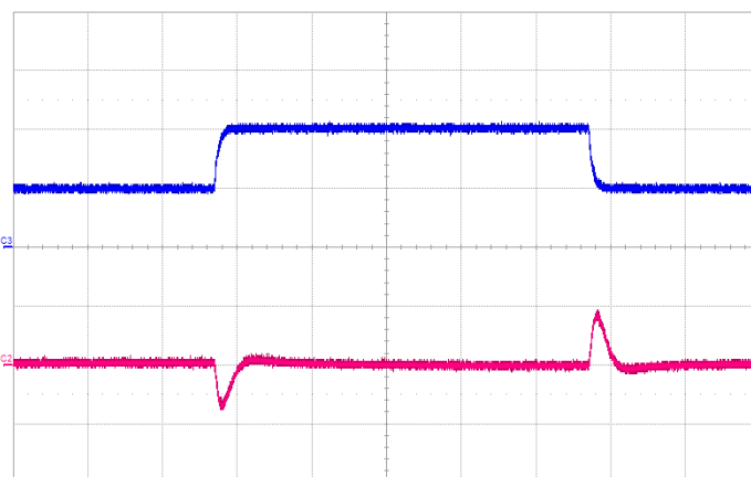
Noise V_{IN}=5V , I_O=10A , 5~20MHz Bandwidth
