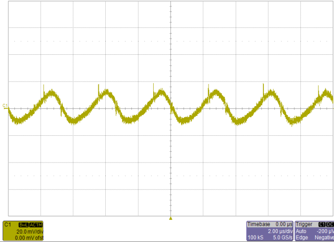
Noise V_{IN}=3.3V , I_O=30A , 5~20MHz Bandwidth
