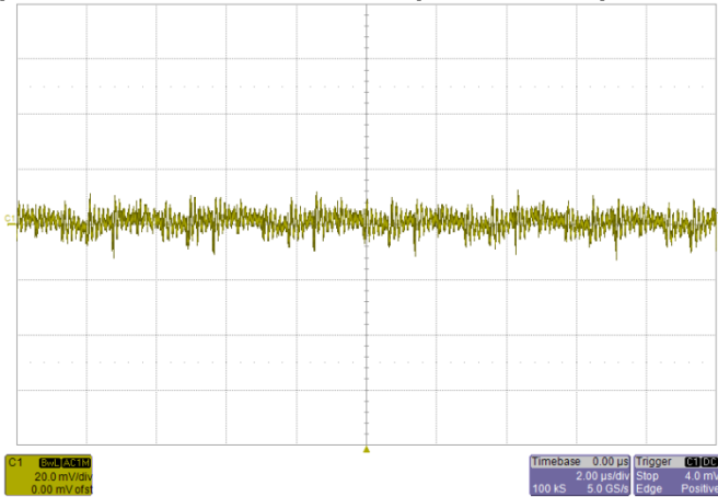
Noise V_{IN}=12V , I_O=100A , 20MHz Bandwidth
