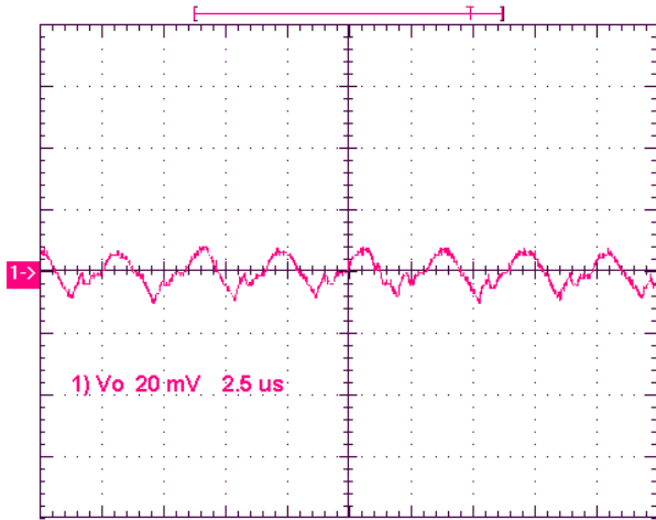
Noise V_{IN}=12V , I_o=5A , 5~20MHz Bandwidth
